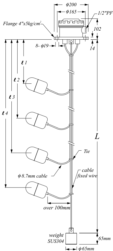
MODEL: FL-A
