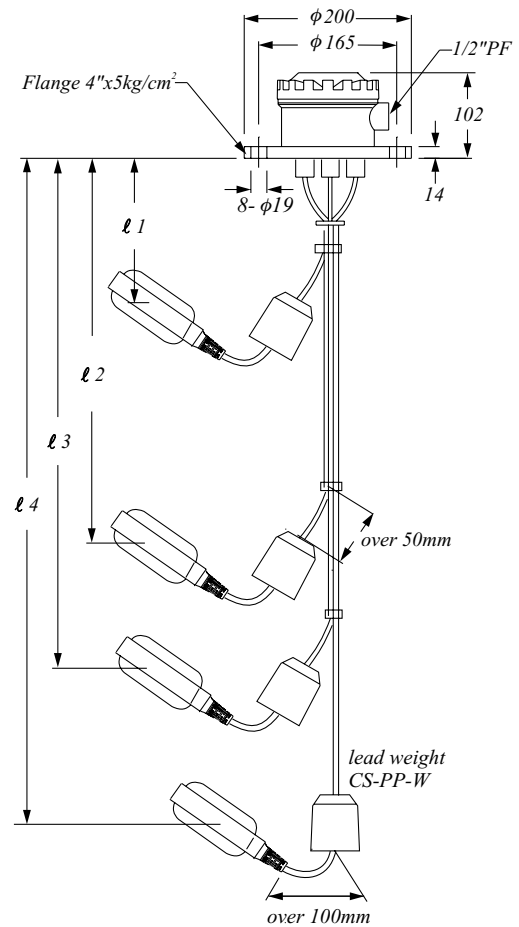
MODEL: FL-B
